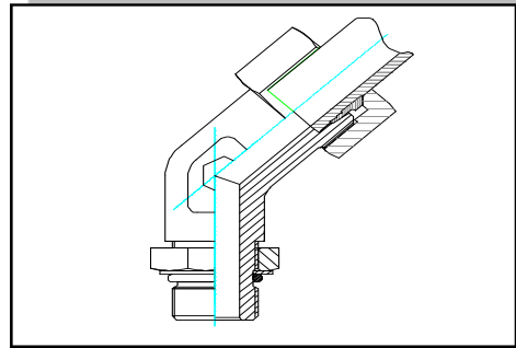
Bulkhead Elbow 45° / R/M/UNF KSD 45° R/M/UNF Kontra Somunlu Dirsek
