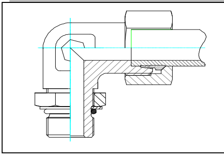
Bulkhead Elbow / R/M/UNF KSD R/M/UNF Kontra Somunlu Dirsek
