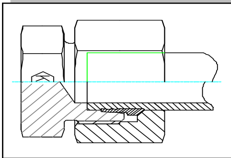
ROV Blanking plug for tube ends BTAP Boru Körleme Tapası
