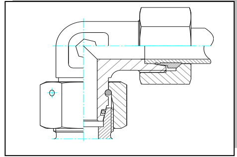
EW Swivel Nut Elbow TD/P Pimli Ters Dirsek
