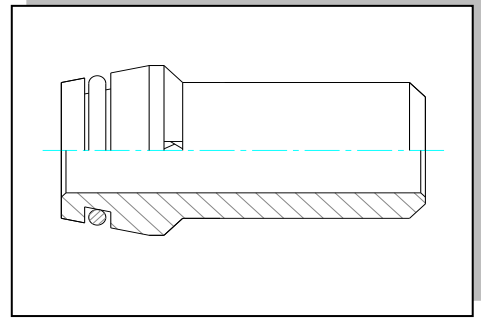
SKA Weld Nipple KY-OR Kaynaklı O-Ringli Yüksük
