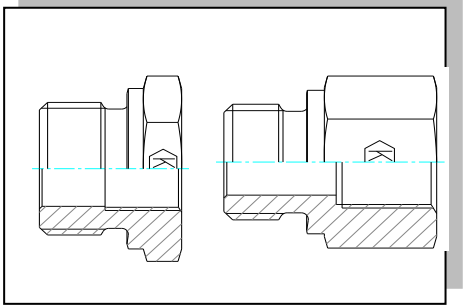
RI Thread Reducer/Expander RD Dişli Redüksiyon
