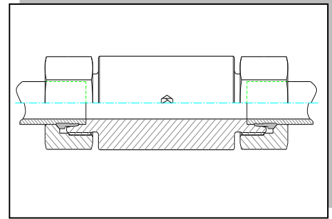
ESV Weld Bulkhead Fittings KPGN Kaynaklı Perde Geçiş Nipeli
