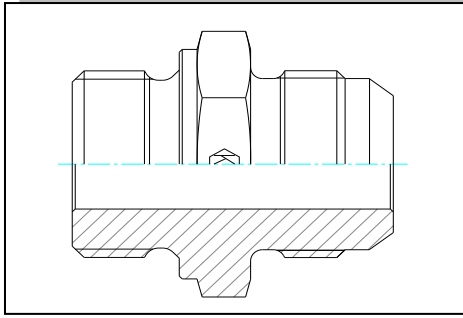
Male Stud Connector JIC 37° HAN Hortum Ara Nipeli JIC 37°
