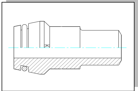
SKAR Reducing Weld Nipple KD/KY-OR Kademeli Kaynaklı O-Ringli Yüksük
