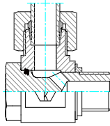
SWVE R/M DD R/M F1
