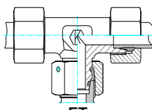
ET OT/P G11
