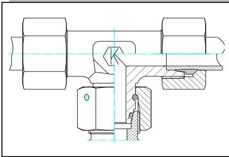
ET Swivel Nut Branch Tee OT/P Pimli Orta Bacak Ters T
