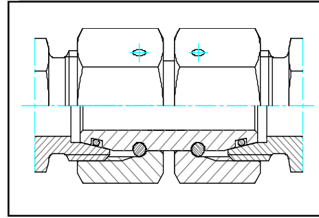
GZ Swivel Union GNP Geçiş Nipeli Pimli
