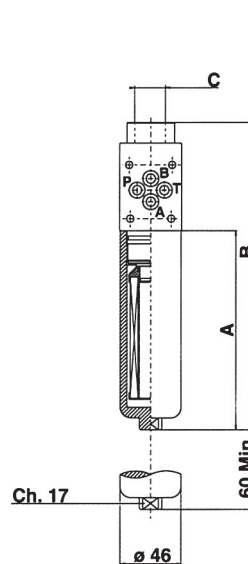
TESTINA CON ATTACCO CETOP 03 HEAD WITH CONNECTION CETOP 03
