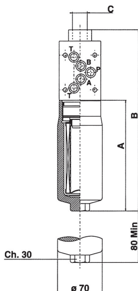
TESTINA CON ATTACCO CETOP 05 HEAD WITH CONNECTION CETOP 05
